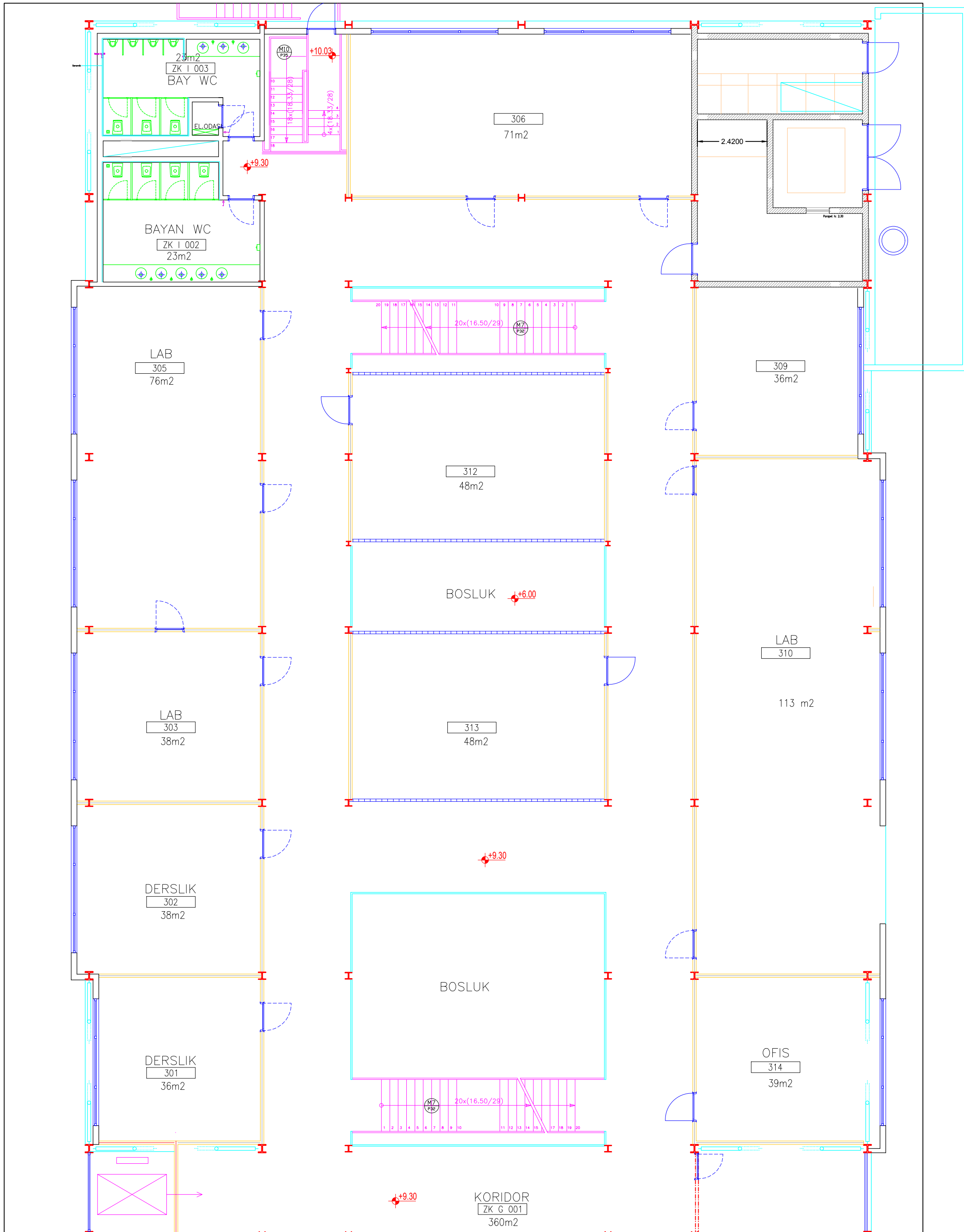
DOLAPDERE_3. KAT PLANI MEVCUT DURUM
