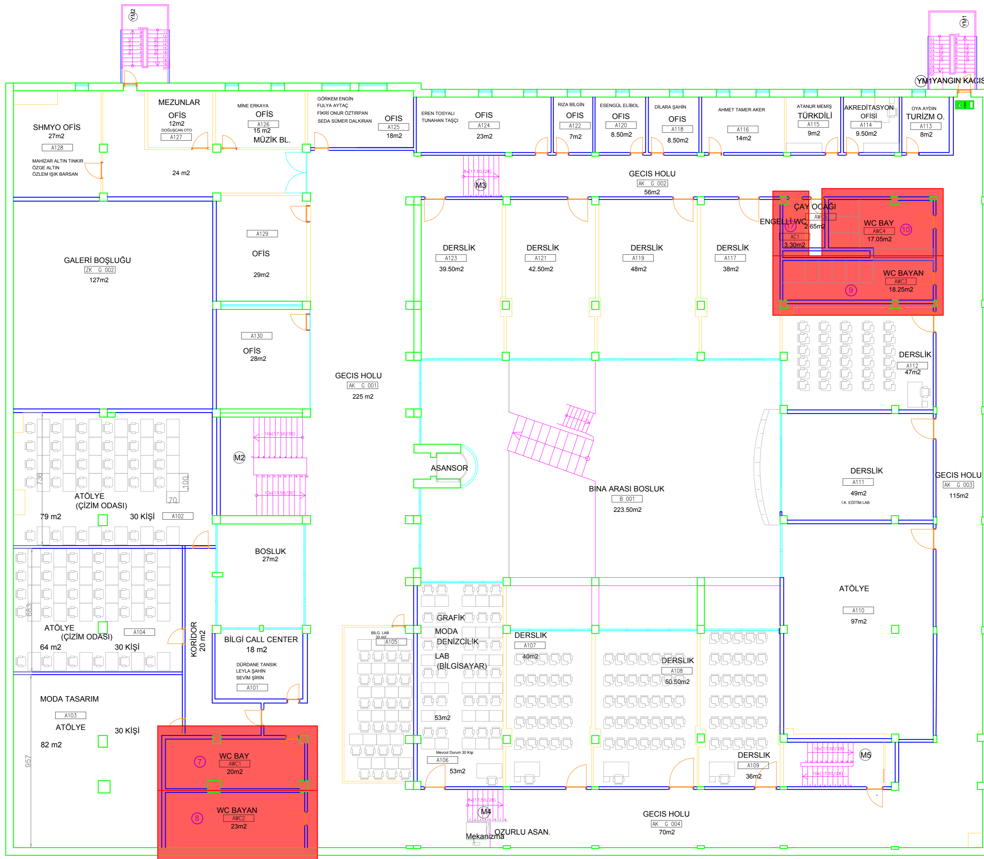
A BLOK 1. KAT PLANI (ESKİ BİNA)
